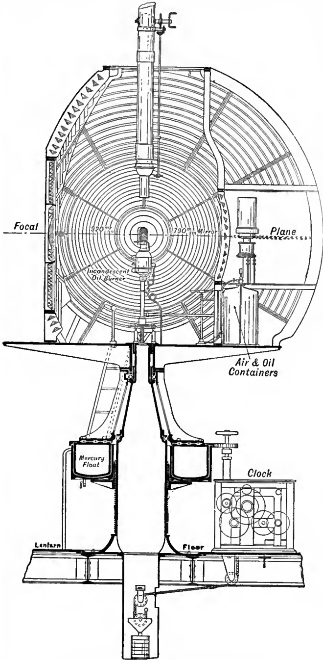
FIG. 42.—Cape Naturaliste Apparatus.
