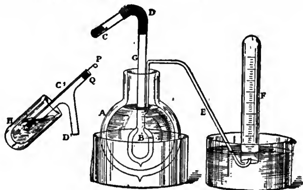
FIG. 13.—Calorimetric Apparatus.
