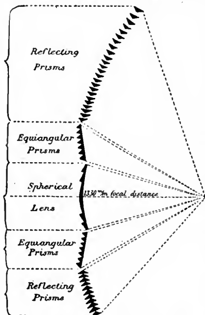
FIG. 40.—Sule Skerry Apparatus.
