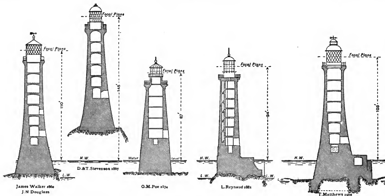
FIG. 14.— Wolf Rock.
