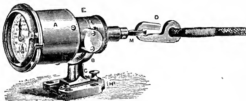
FIG. 4.—The Cherub Log.
