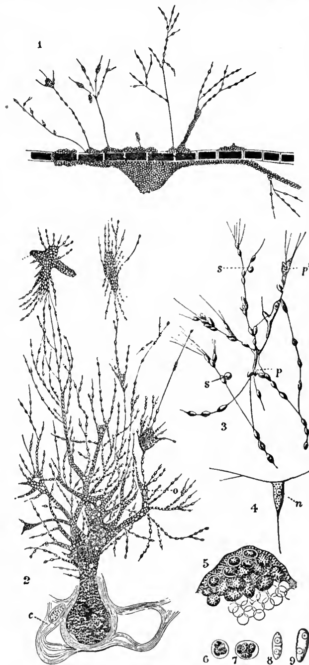
Labyrinthulida.
