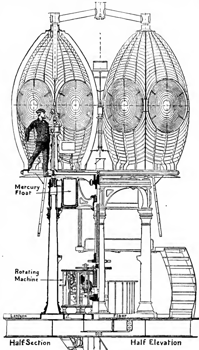
FIG. 43.—Île Vierge Apparatus.
